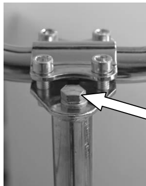
(c) Rozpínací šroub
