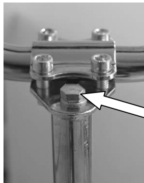
(c) Rozpinacia skrutka
