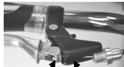
Oválny koniec brzdového lanka
